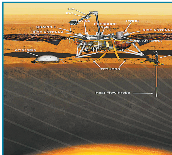
▼12月22日,美国宇航局宣布,因技术原因,将推迟原定于2016年3月InSight火星探测器的发射。图为InSight火星探测器探测火星深处的概念图。
