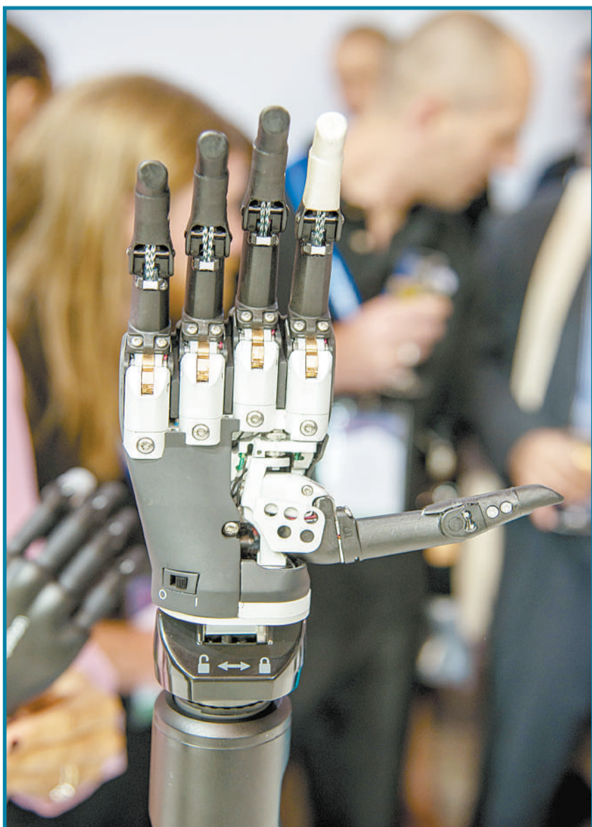
6月22日,法国里昂,仿生用品制造商向媒体展示拥有五个指头的仿生机械手,该仿生义肢是首个被法国健康系统认可的产品。
