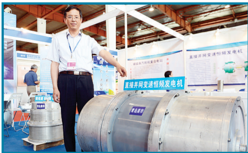
美华永磁电机科技有限公司制造的世界首台可直接并网的变速恒频发电机。
