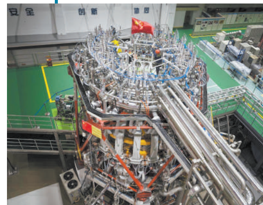
1984年,中国环流器一号(HL-1)的建成,被认为是我国核聚变研究史上的重要里程碑。图为新一代“人造太阳”(HL-2M)装置。
