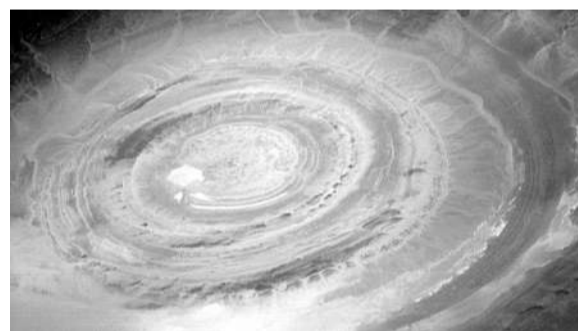
这个位于撒哈拉沙漠中的巨大同心圆地形被称为“理查特结构”,直径达50公里,是一个严重侵蚀形成的地质结构。
