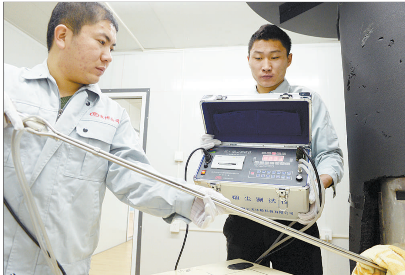
河北霸州京博公司“β传感器式快速烟尘测试仪”的问世,颠覆了30年来传统的滤筒称重检测烟尘的方法,检测效率和准确率均大幅提高,也填补了我国在这一领域的技术空白。
